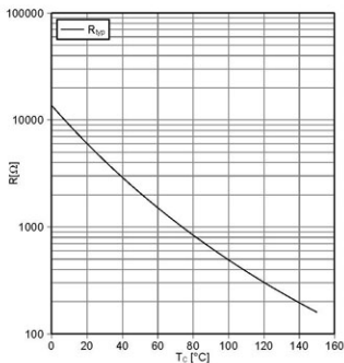
NTC-Widerstand-Temperaturkennlinie (typisch) NTC-Thermistor-temperature characteristic (typical) R = f(T)
